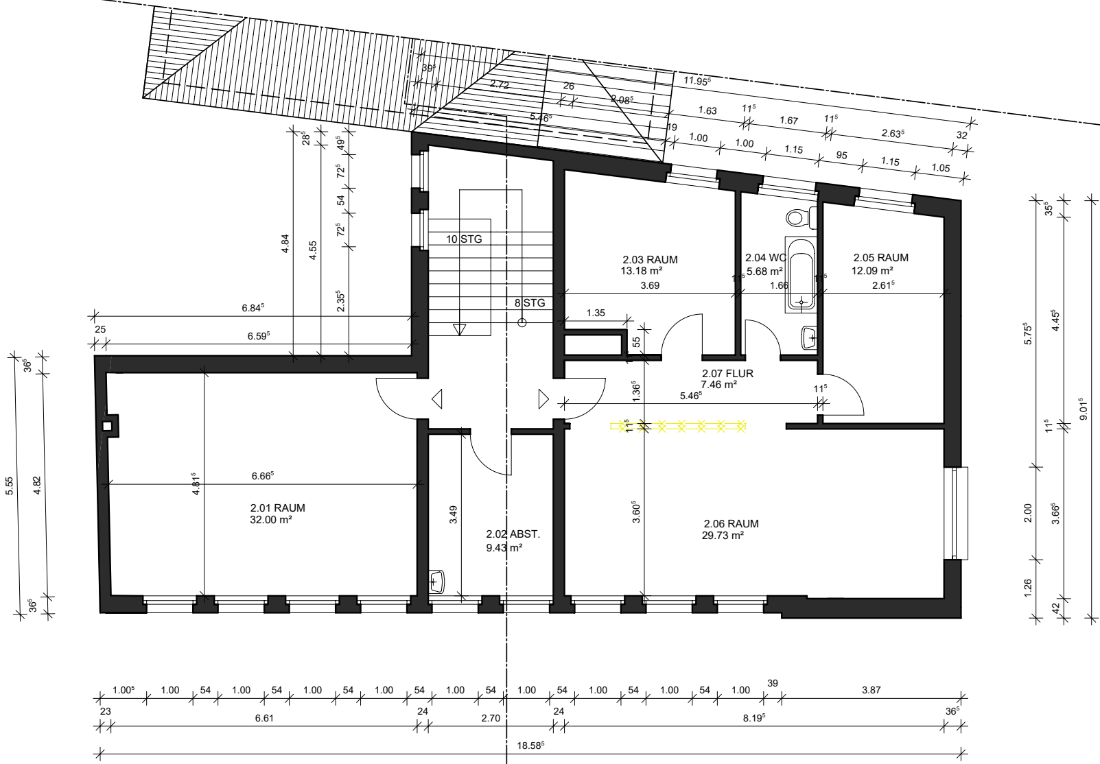
Grundriss 2.OG
