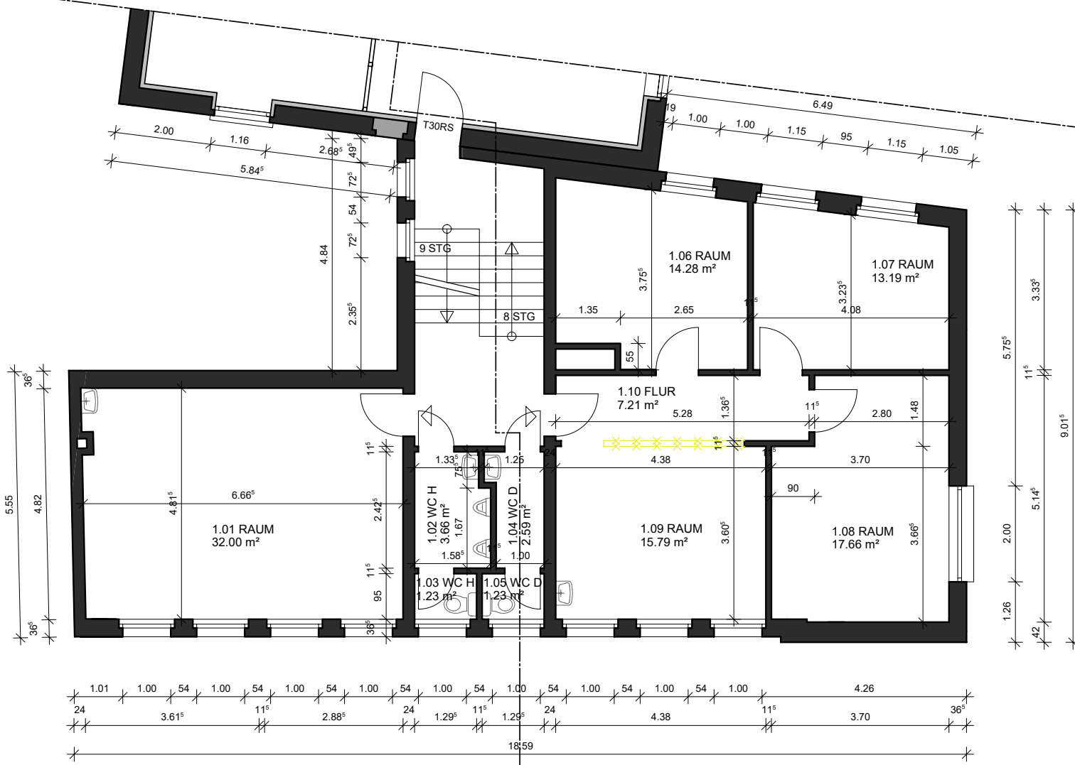
Grundriss 1.OG
